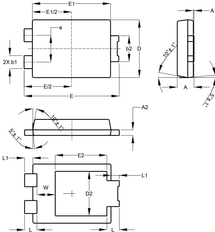
PowerDI5
